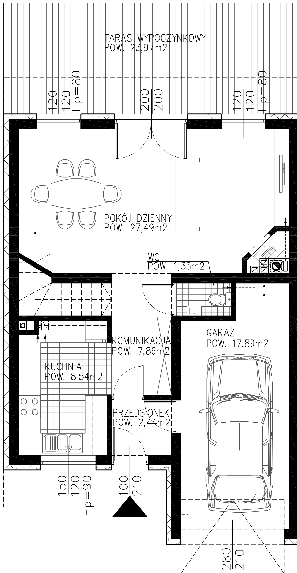
RZUT PARTERU
