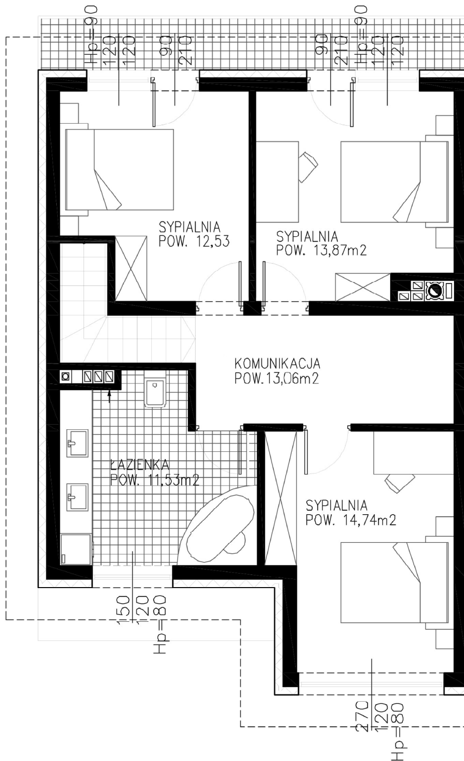
RZUT I-go PIĘTRA
